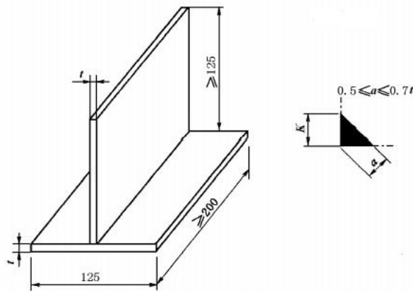
图2 板材角焊缝试件
