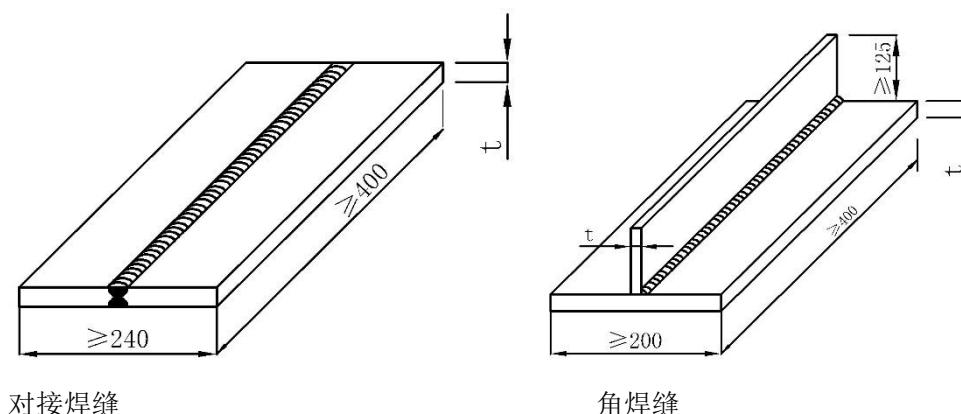
图4 焊接操作工操作技能评定试件
