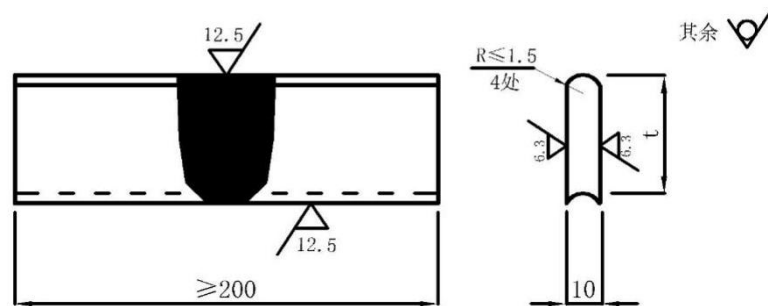
b) 侧弯试样
