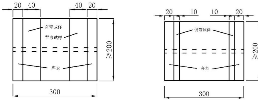
图5 板材试件取样位置
