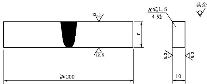
a) 面弯、背弯试样
