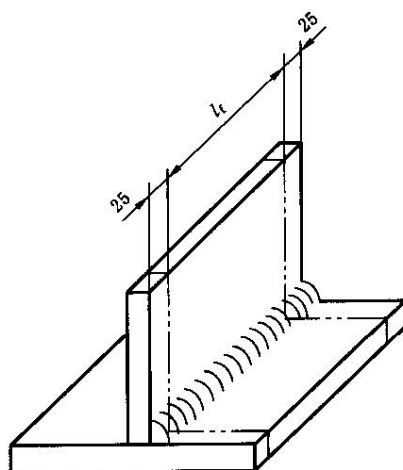
图9 板材角焊缝的试验长度
