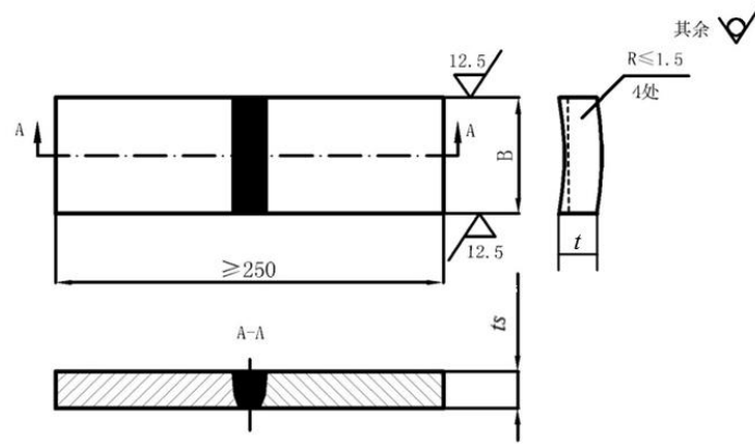
a) 面弯、背弯试样
