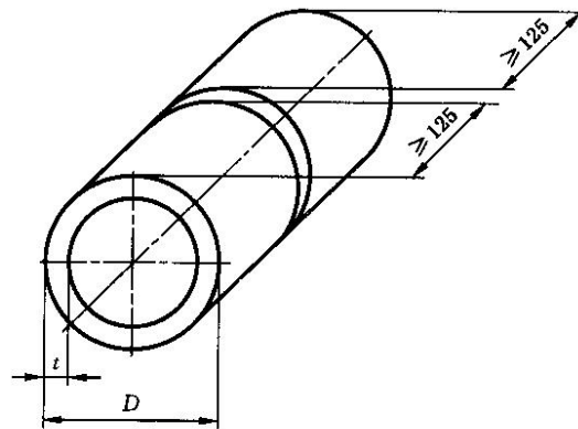
图3 管材对接焊缝试件
