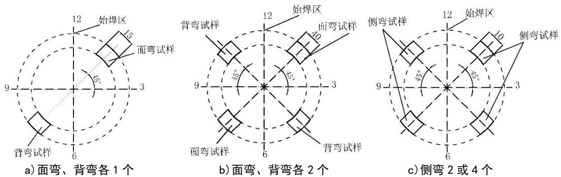
图7 管材试件取样位置
